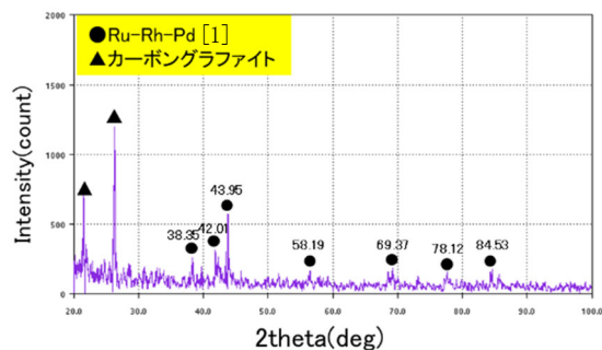
図 1 Ru-Rh-Pd 合金における XRD パターン
