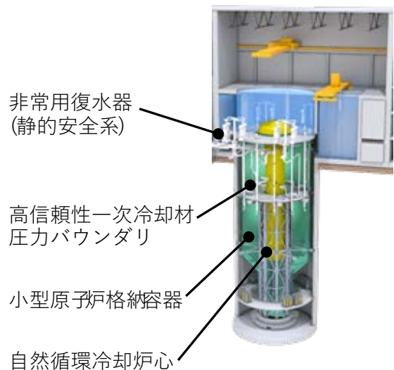
図 1 BWRX-300 の概念図
