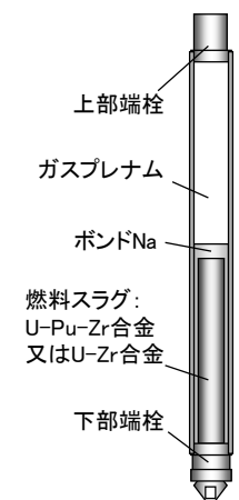
図2 金属燃料ピン
