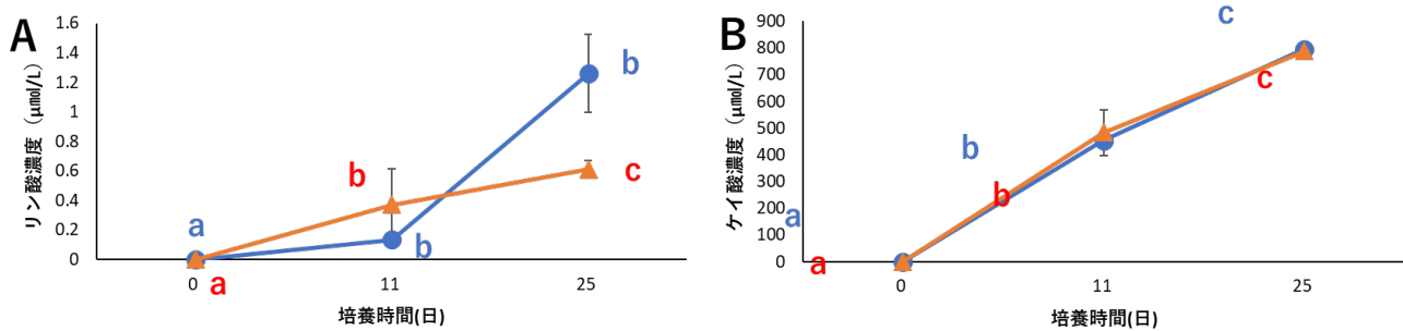
Fig.1 瓶実験による土壌母材の無酸素条件下の炭酸風化に伴う濃度変化
