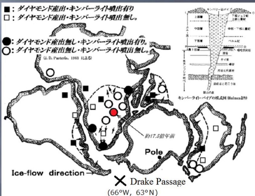
図. 3 Ice-flow directions, palaeomagnetic pole position and extent of Late Carboniferous glaciations. キンバーライト・パイプ(噴出)と、ダイヤモンド産出状況
