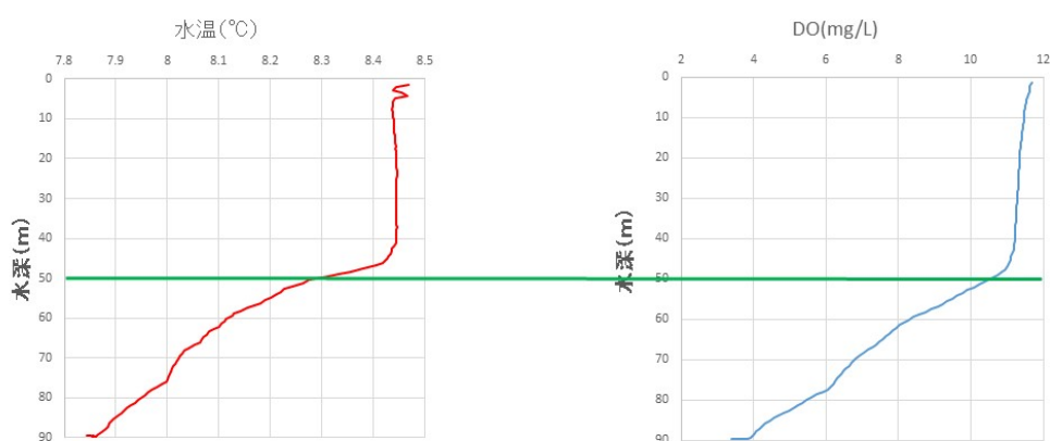
琵琶湖北湖第一湖盆での水温と溶存酸素濃度(2019年3月24日) 水深50m以深が混合していない！
