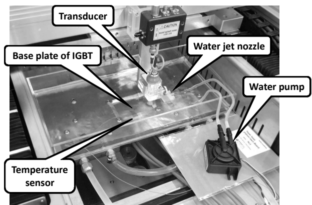
Fig. 2 DUT Setup
